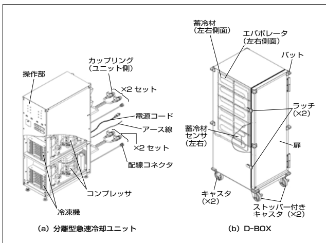
図3 内部構造
