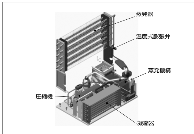
図4 冷凍機の構造
