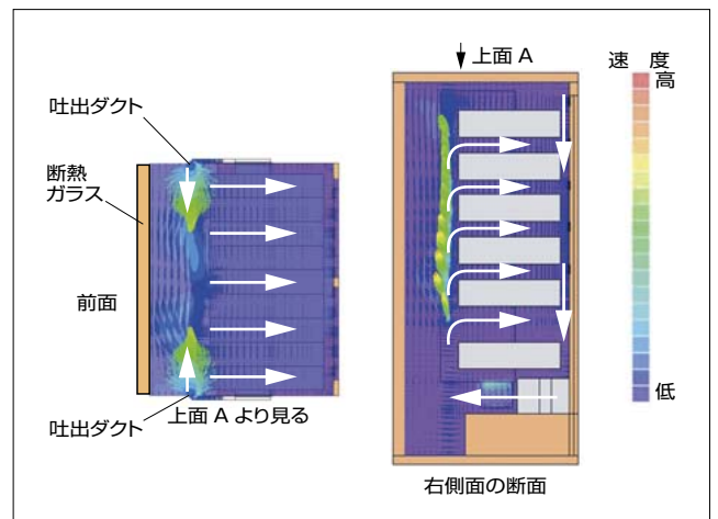
図 5 風の流れの設計とシミュレーション結果（従来構造）
