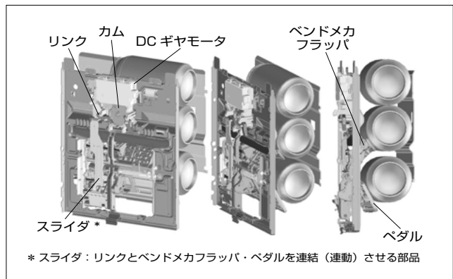
図2 ベンドメカ
