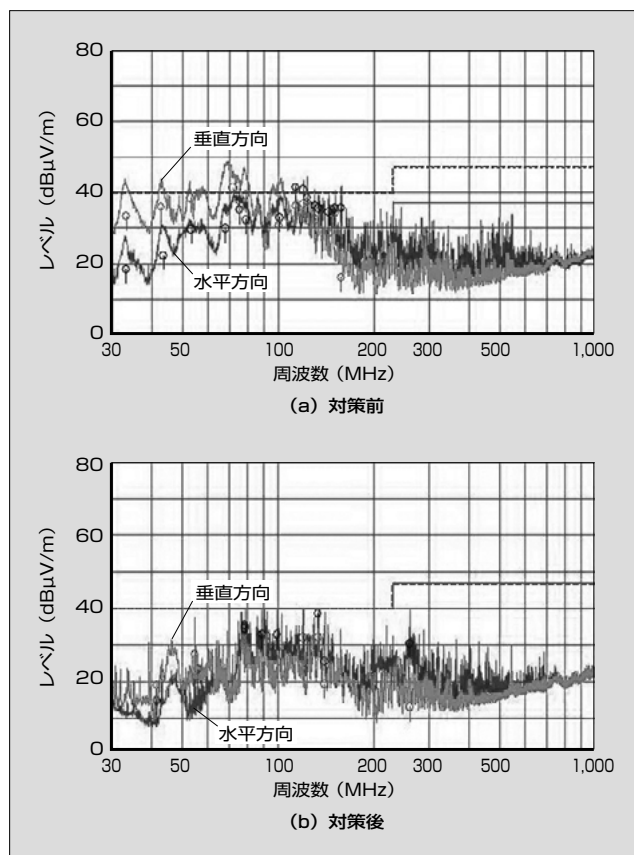
図9 自動販売機の放射エミッション
