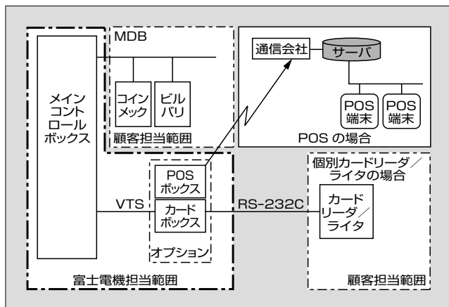
図8 金銭処理部の構成
