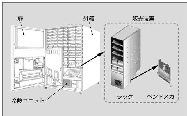
図1 自動販売機の製品構成
