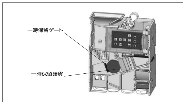
図4 アクセプタユニット(正面カバーを外した状態)
