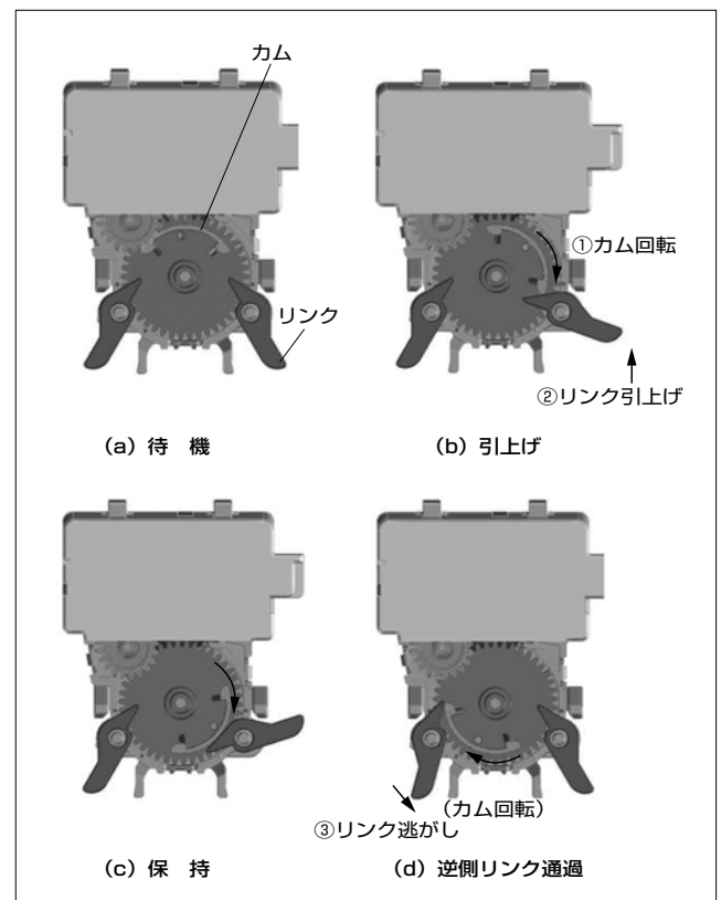
図4 駆動源の動作
