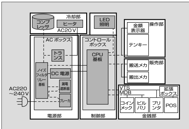
図7 制御システムの構成
