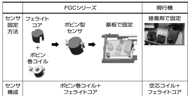
図3 検銭センサの構成
