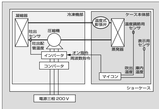
図3 冷凍機システムの構成
