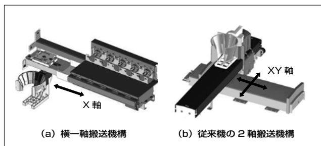
図7 搬送機構
