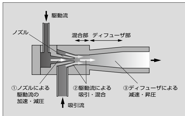
図1 エジェクタの動作
