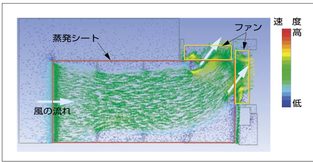
図8 気流解析結果
