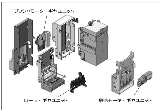
図8 保守部品ユニット構造
