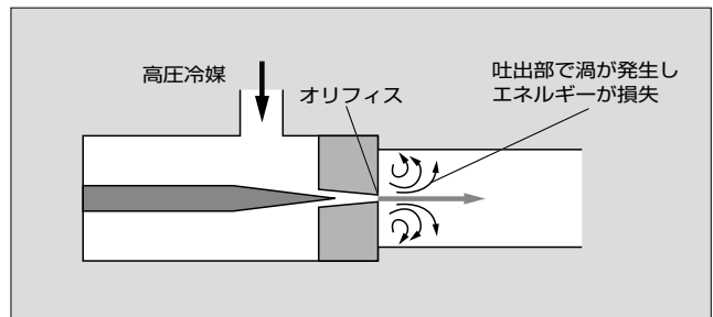
図2 従来の膨張弁における渦の発生
