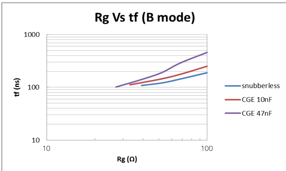
CGE 有無による tf のゲート抵抗依存性
