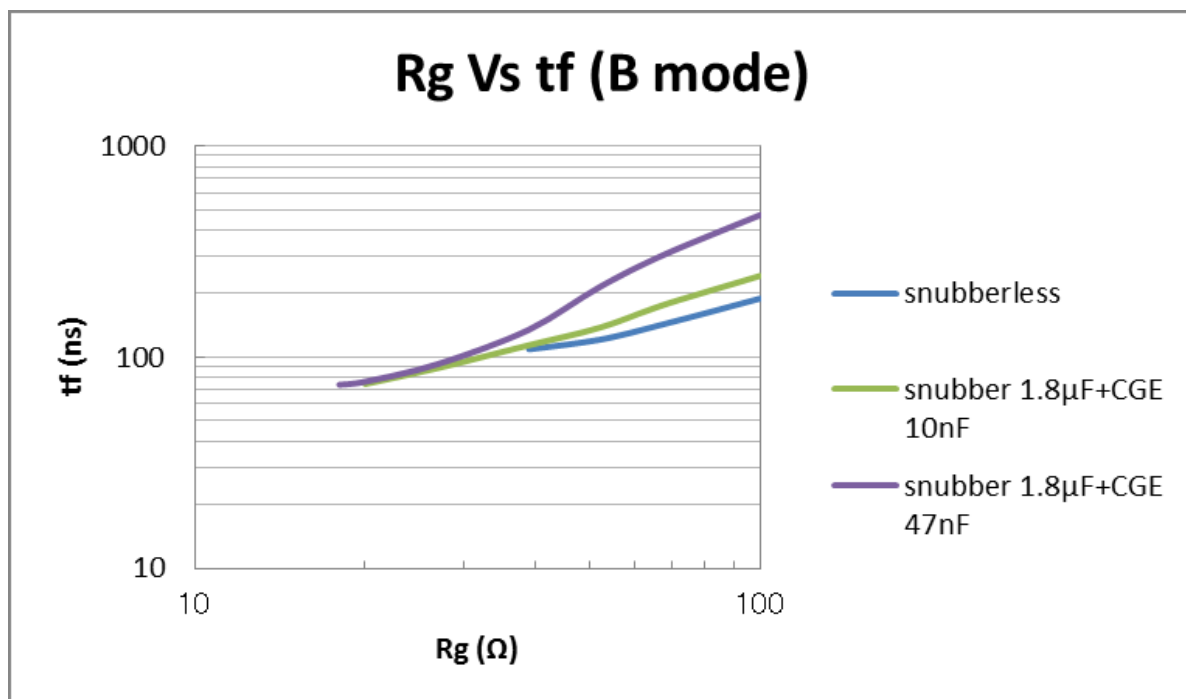
スナバ及び CGE 有無による tf のゲート抵抗依存性
