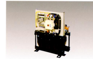
リアクトル始動器 [ブランド名: 電光工業(株)] Reactor starters
