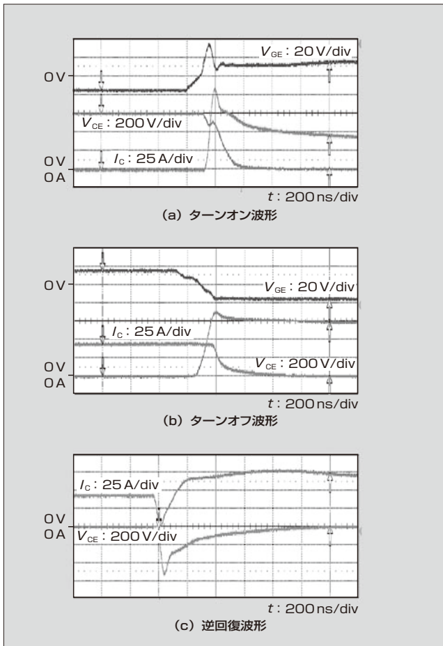
図2 スイッチング波形 (「7MBR35VKD120-50」)
