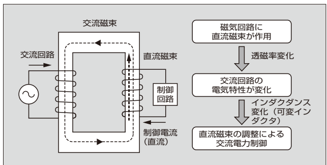
図 3 他励式配電系統用 SVC の基本原理
