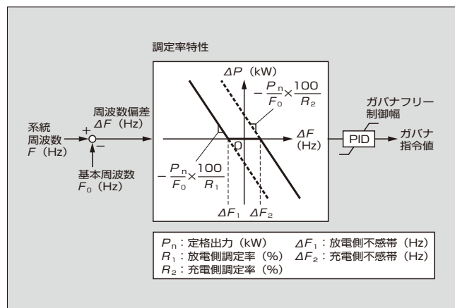
図 4 ガバナフリー相当制御の制御ブロック
