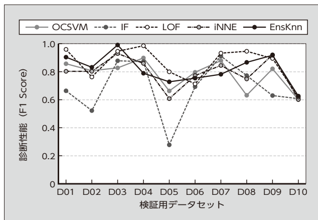
図4 機械学習手法による診断性能の比較
