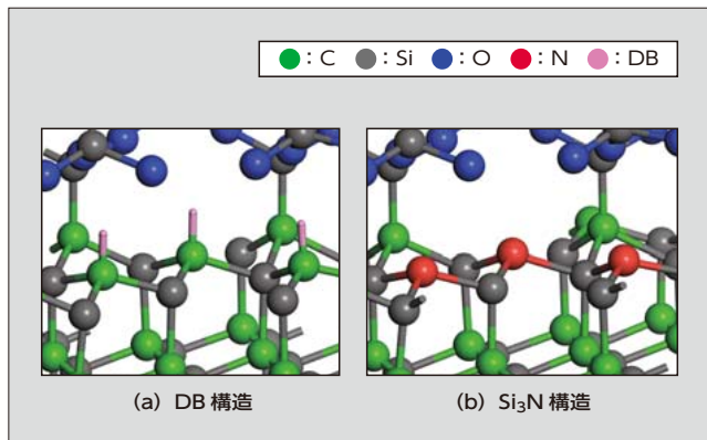
図5 SiC/SiO 2 界面の DB 構造と \text{Si}_3\text{N} 構造のモデル図
