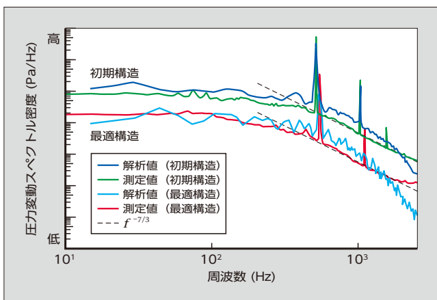
図8 ファンの下流の壁面に作用する圧力変動スペクトル
