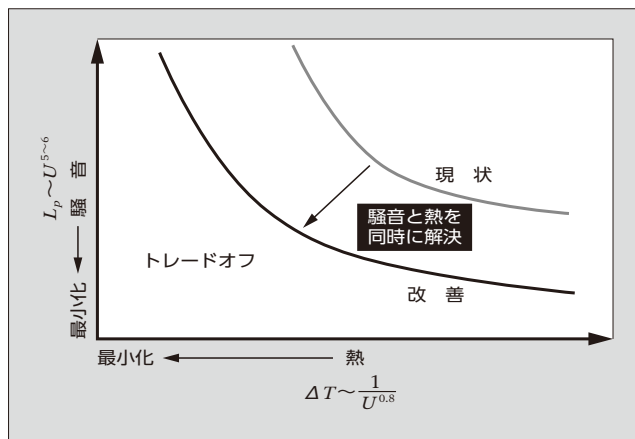
図3 製品設計における流体騒音と温度の関係
