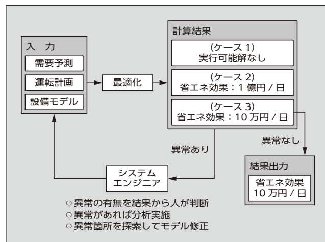
図7 従来のエンジニアリング
