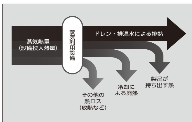
図 1 蒸気利用設備の熱収支関係
