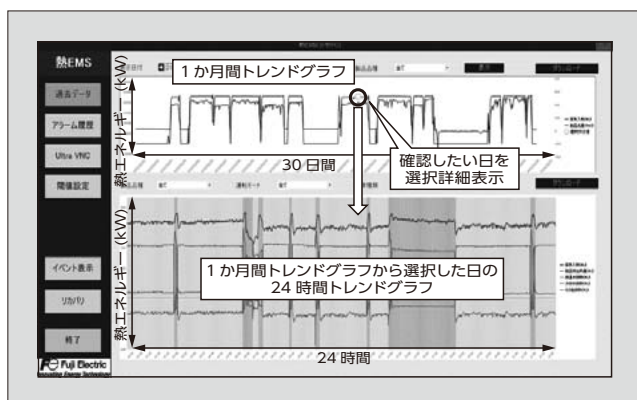
図6 過去データ検索画面
