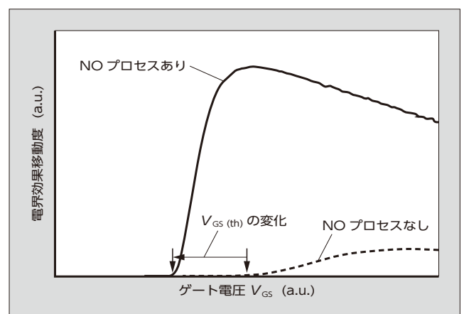
図 4 SiC-MOSFET の移動度特性の例
