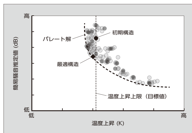
図 5 多目的最適化による検討結果
