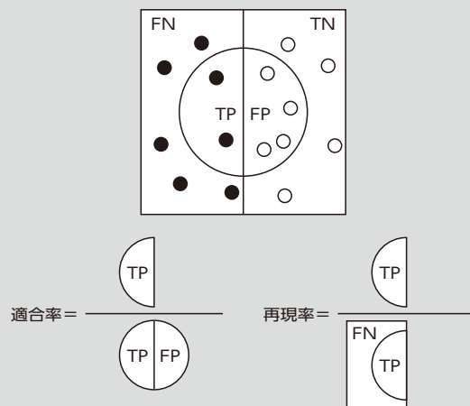
図 6 テキスト認識技術の認識精度計算方法
