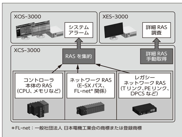
図2 RASの構成
