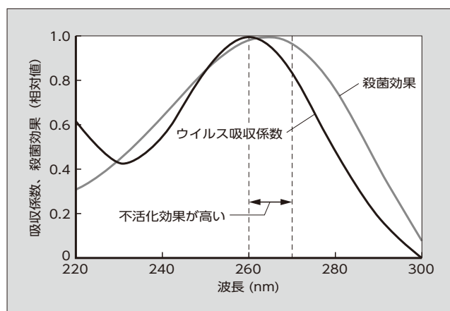
図 1 ウイルスの紫外線吸収係数と殺菌効果 (5)(6)
