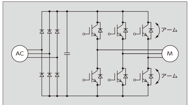
図1 スwitchング回路
