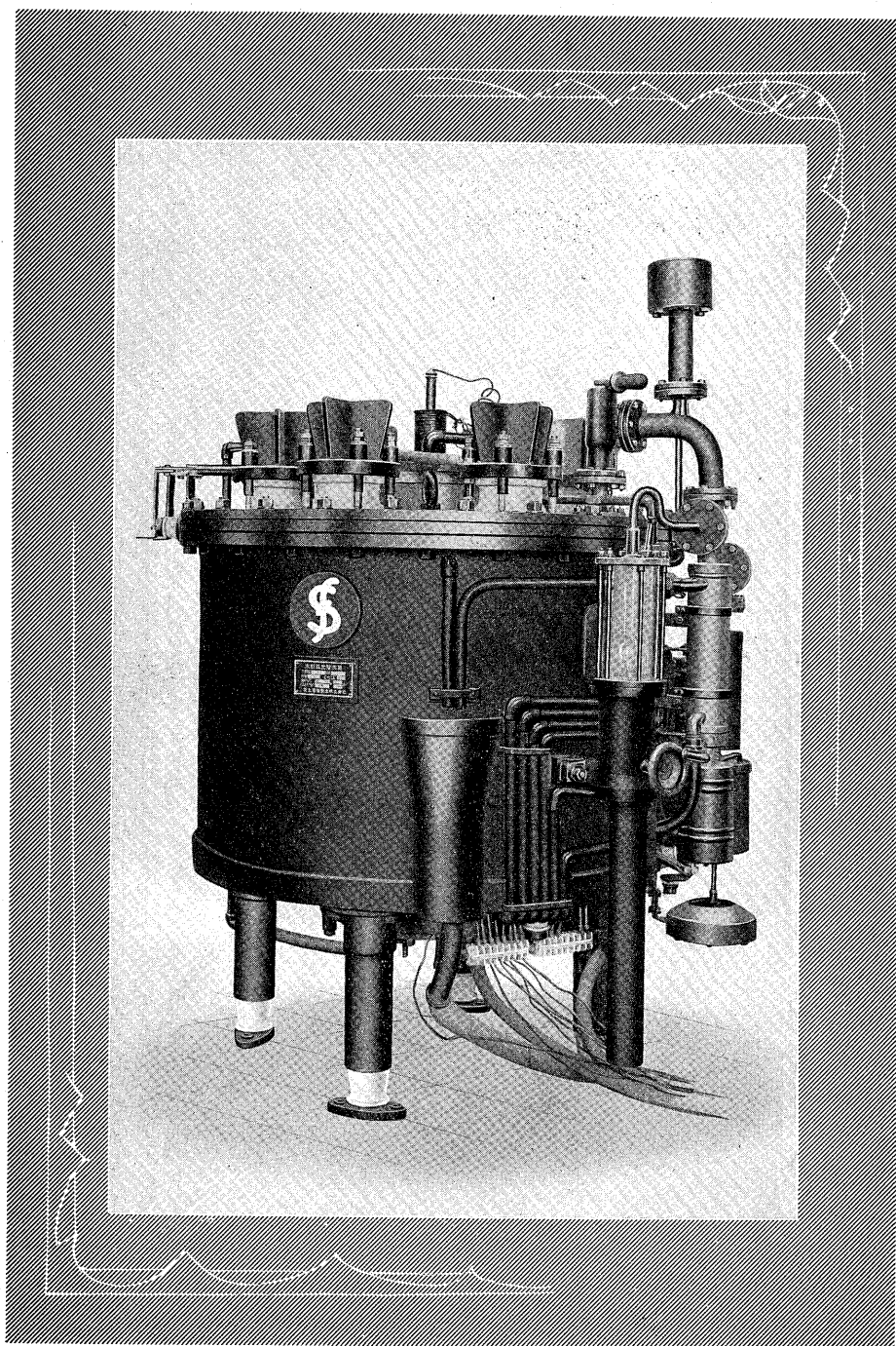
新型富士水銀整流器 500KW. 600V. 50% 2時間過負荷 (静岡電鐵株式會社納品)
