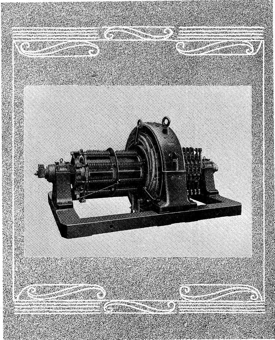
旭電化株式會社納入 富士廻轉變流機 1700/1200KW—425/300V—50 \sim 750r.p.m 型 DUG 440/28
