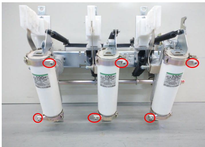
○部 ヒューズクランプ取付ねじ、6ヶ所
