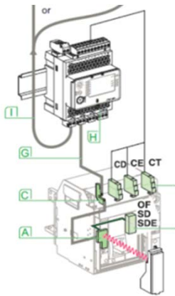
IO Module + Masterpact NT/NW / Compact NS630b-3200 / PowerPact P-, R-Frame
