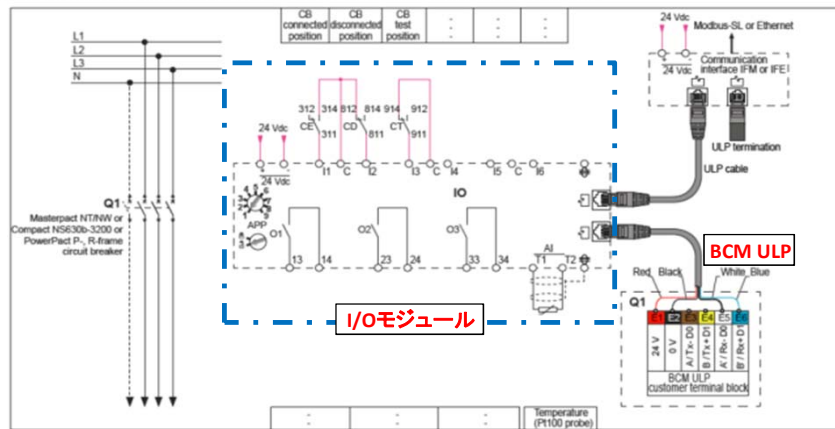
IO Module + Masterpact NT/NW / Compact NS630b-3200 / PowerPact P-, R-Frame
