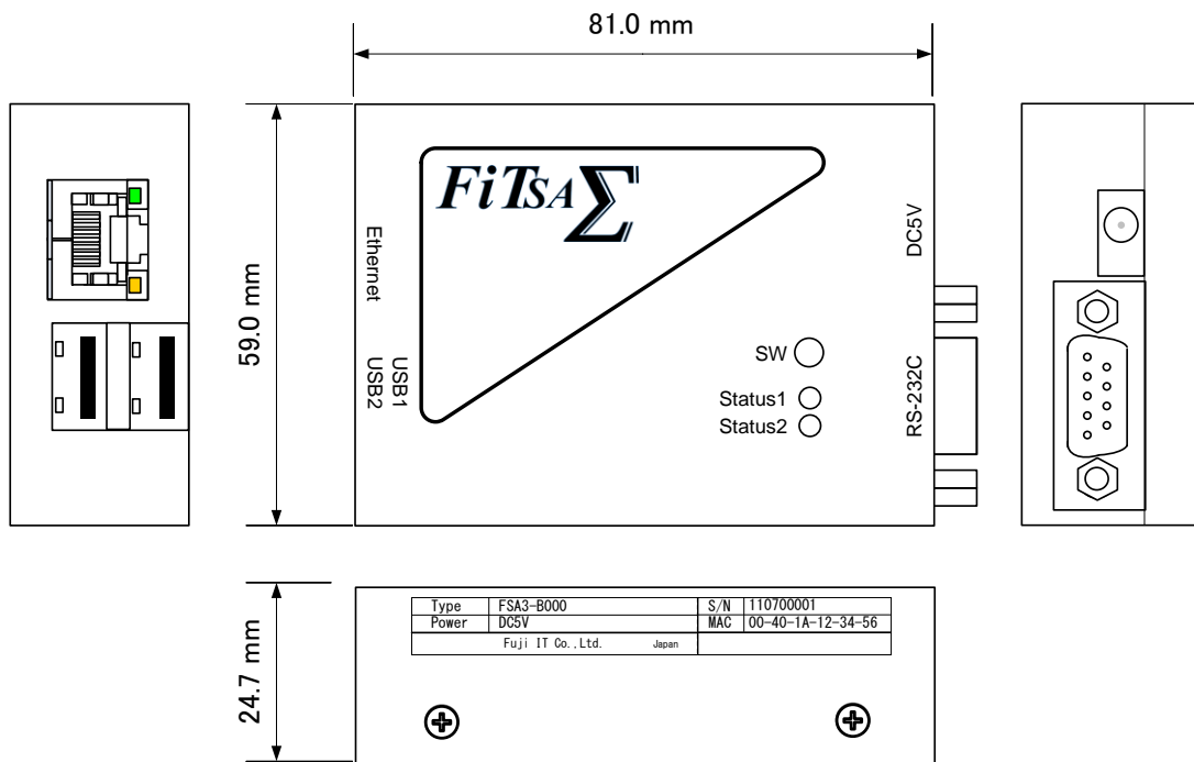
本体前面・側面図
