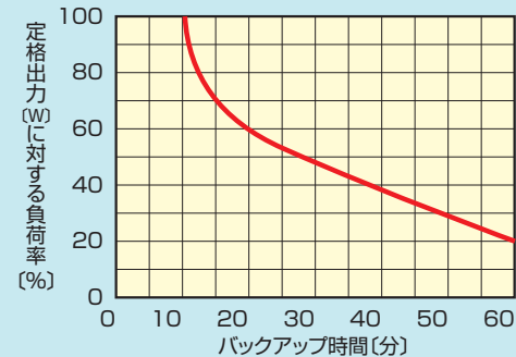
バッテリーバックアップ時間(標準バッテリーの場合)
