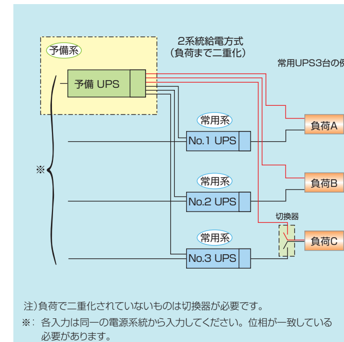
待機冗長システム(簡易二重化)N+1システム
