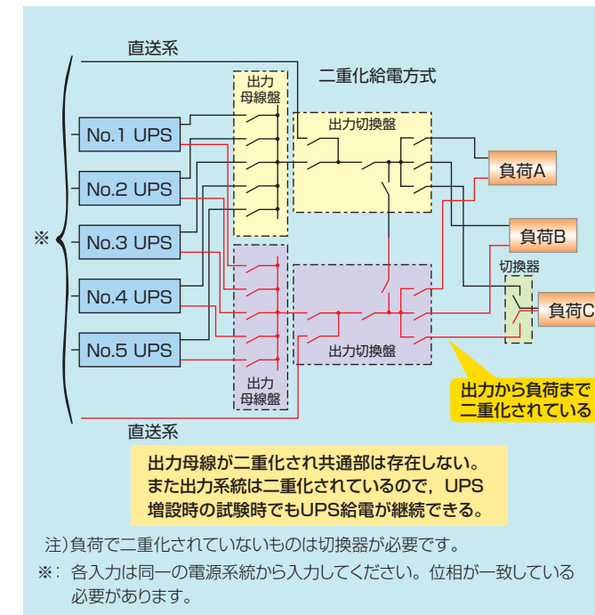
並列冗長システム(簡易二重化)N+1システム
