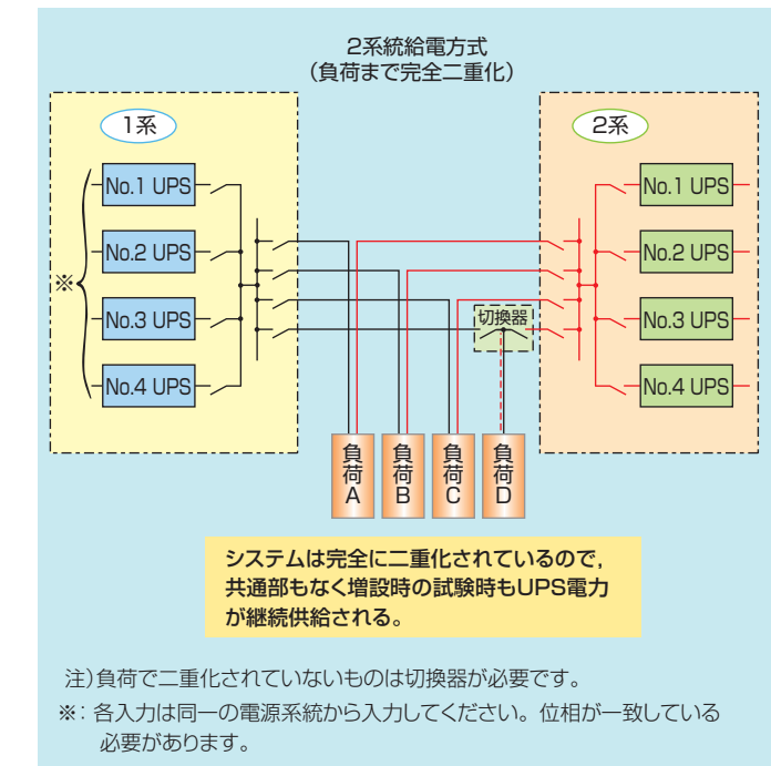
並列冗長システム(完全二重化)2Nシステム
