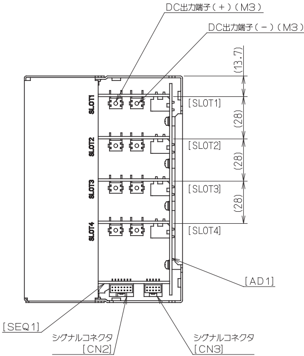
VIEW P (底面から見る)
