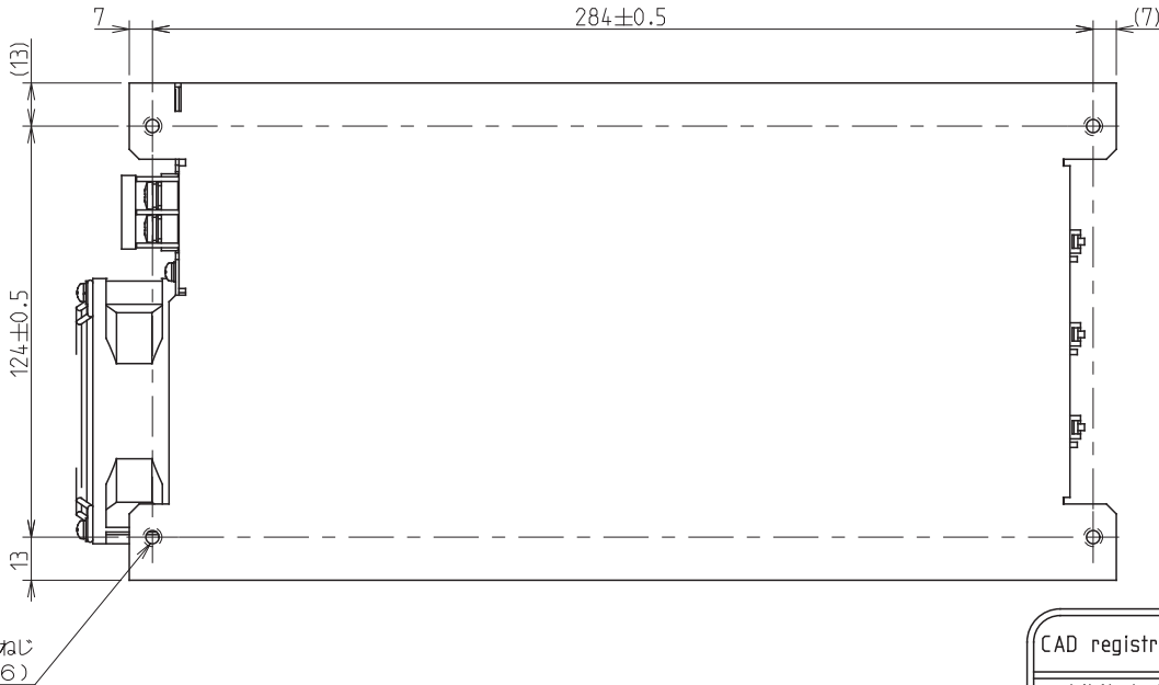
VIEW P (底面から見る)
