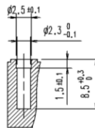
図 2(d) 断面
