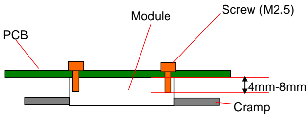
図 2(a) ネジによるモジュールへの PCB の取り付け
