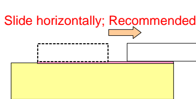
図 6 ネジ止め後の取り外し工程の一例
