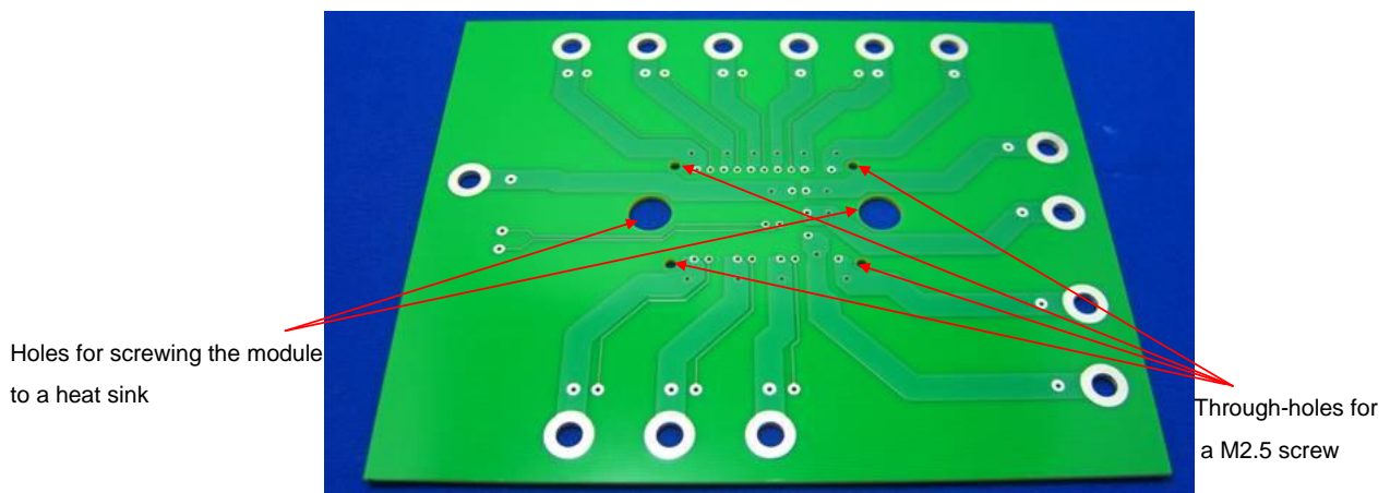
図1 PCBの一例
