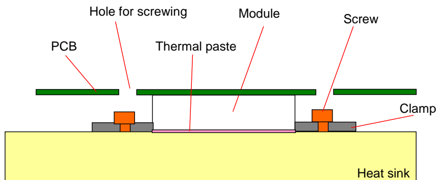
図 5(a) ヒートシンクへのモジュールの実装
