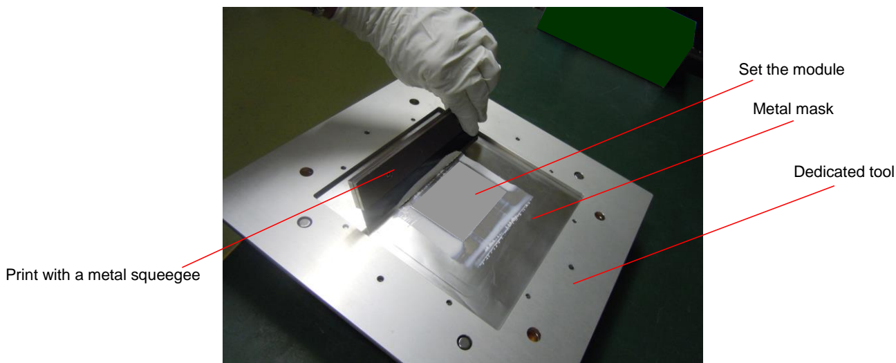
図4 ステンシルプリント工程
