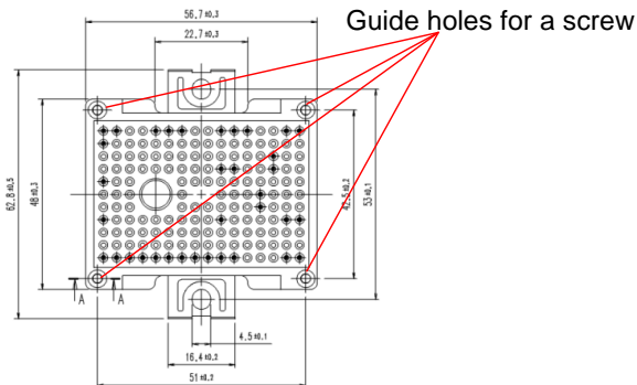
図 2(c) ネジ用ガイド穴(2B)
