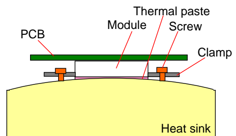
図 3(b) ヒートシンクの平坦度
