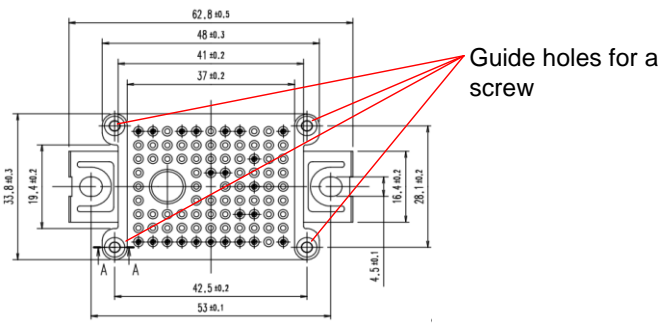
図 2(b) ネジ用ガイド穴(1B)
