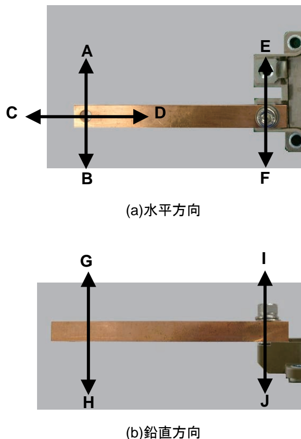
図2 印加応力方向を示した図
