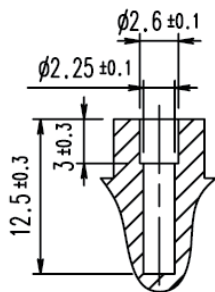
(a) PCB 取り付け用穴
