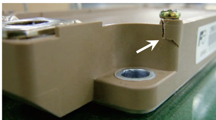
図 7 推奨ネジ以外でとりつけた場合のモジュール破損
