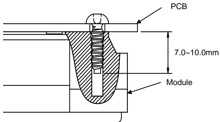
図5 中央部、コーナー部のネジ取り付け時の断面模式図
