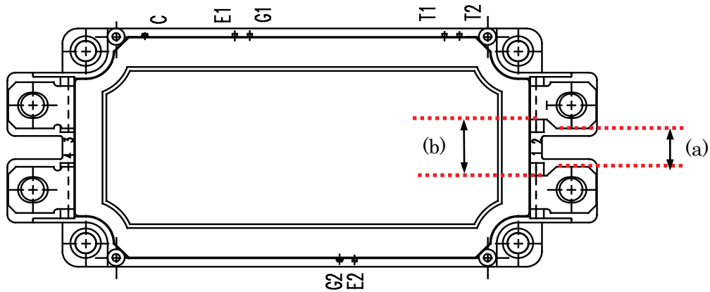
図 3 IGBT モジュールの主端子に対する空間距離と沿面距離
