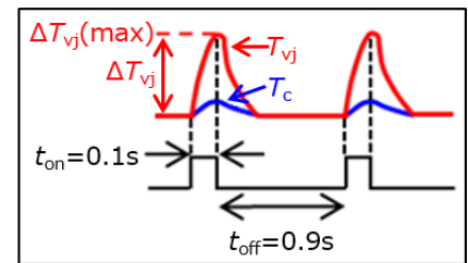
\Delta T_{vj} パワーサイクル試験波形
