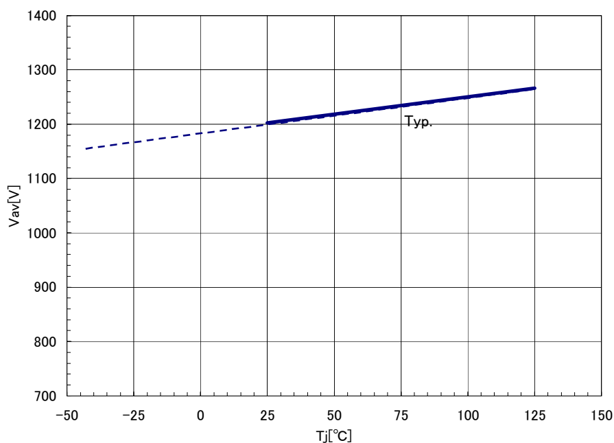
2MBI300U4H-120
