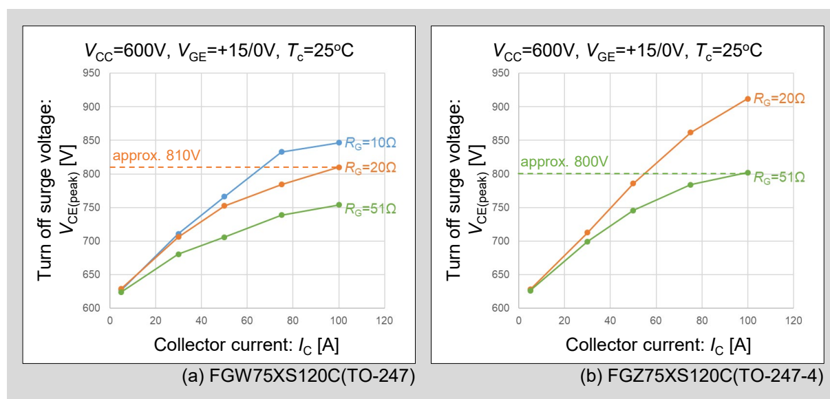
図3-4 ターンオフサージ電圧比較
