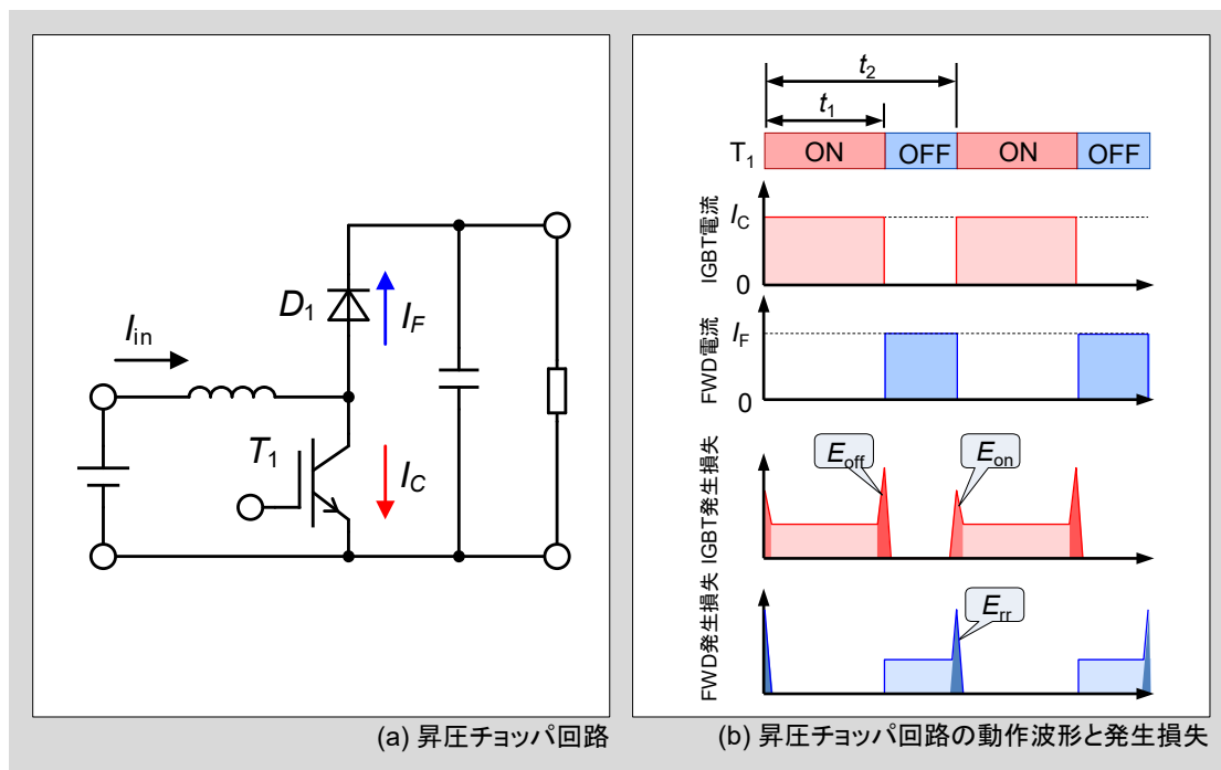
図6-4 昇圧チョッパ回路での発生損失
