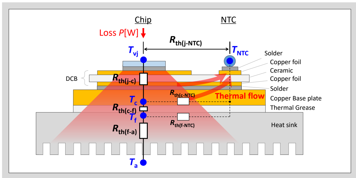
図2. 熱モデルの概念図
