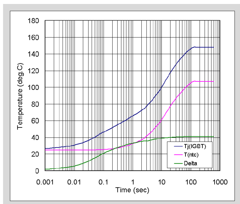
図4. 接合温度とサーミスタ温度の時間応答性
