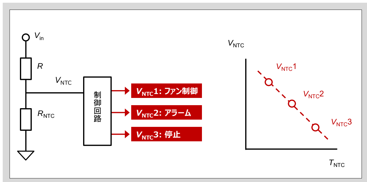
図5.温度検出回路の一例
