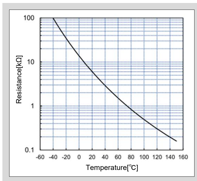
図3. NTCサーミスタの温度特性
