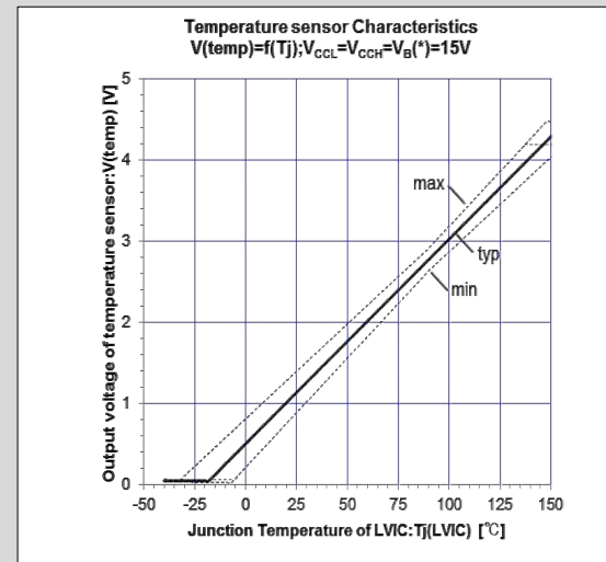
図3-25 LVIC温度とTEMP出力電圧特性 プルダウン抵抗:22kΩ
