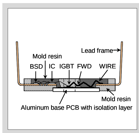
図1-3 パッケージ断面構造
