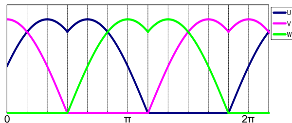
変調波 (2 相変調)
