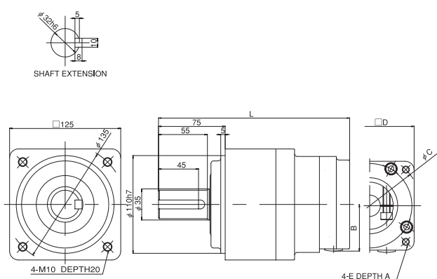
外形図 4
