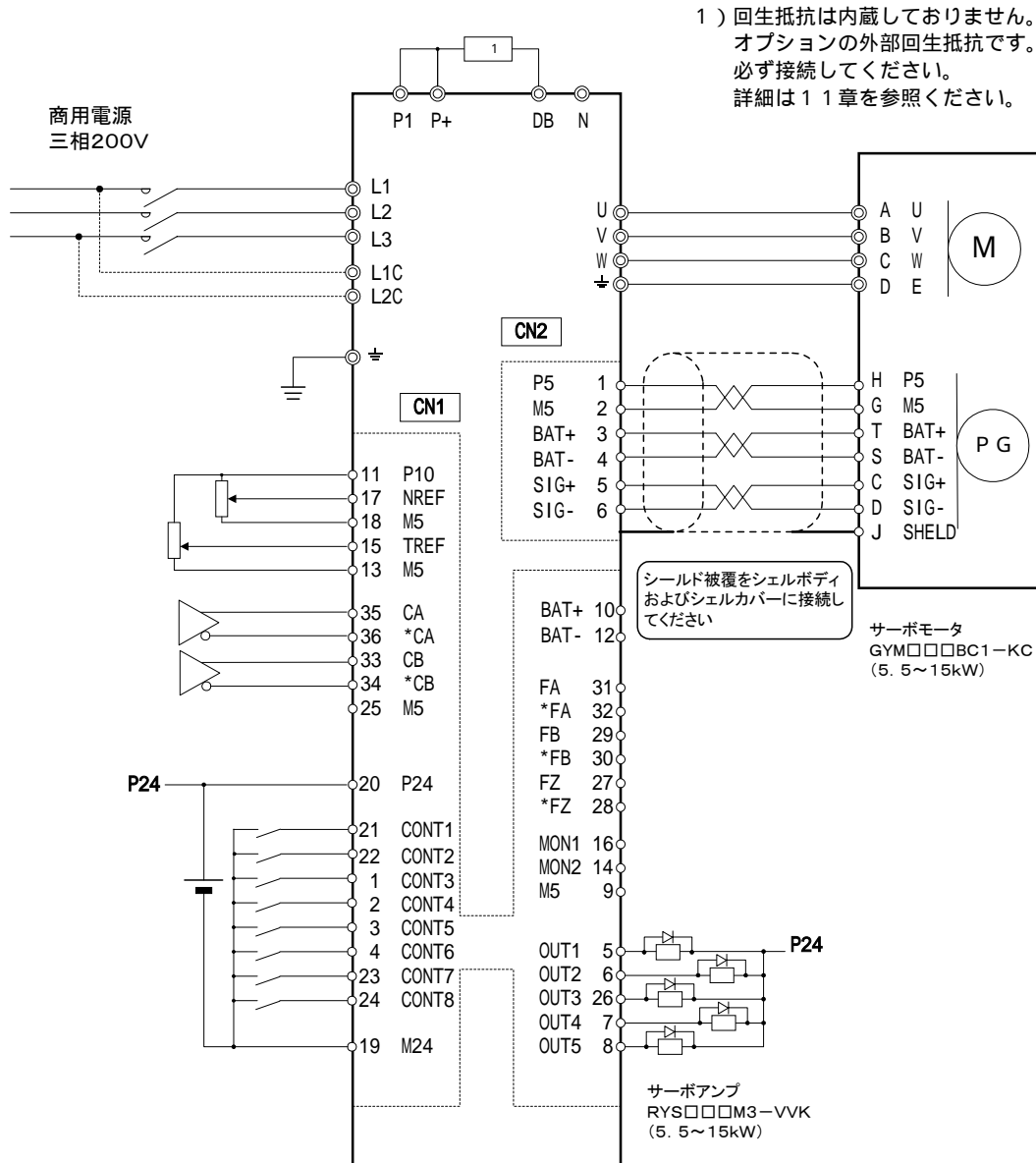
標準接続図(中容量:5.5~15kW)
