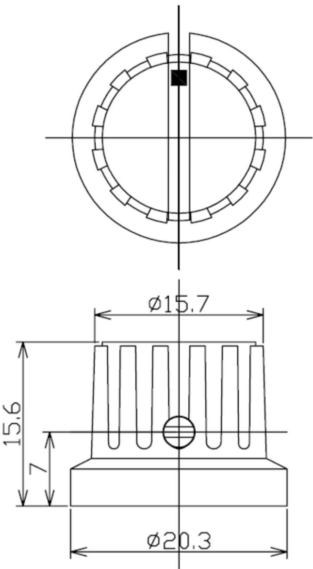
固定ねじ M3 すりわり付きねじ
