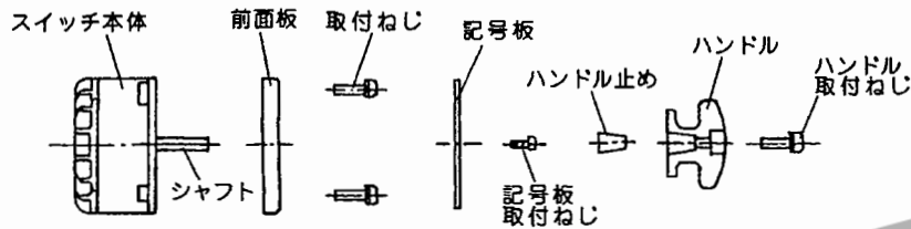
第3図 スイッチの取付方法
