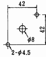
第2図 取付穴明図(42mm)
