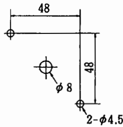
第1図 取付穴明図(48mm)
