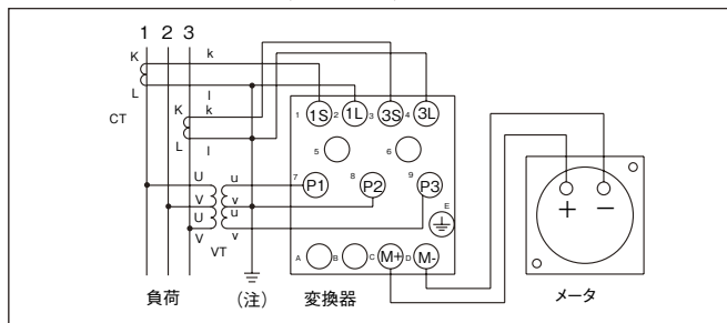
図2 三相不平衡力率計 (三相3線) FR-□ PFU形、WM8A26形
