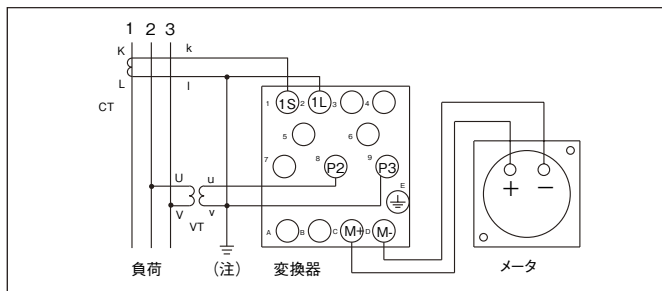
図1 三相平衡力率計 (三相3線) FR-□ PF3形
