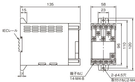
図1 三相平衡力率計 (三相3線) FR-□ PF3形
