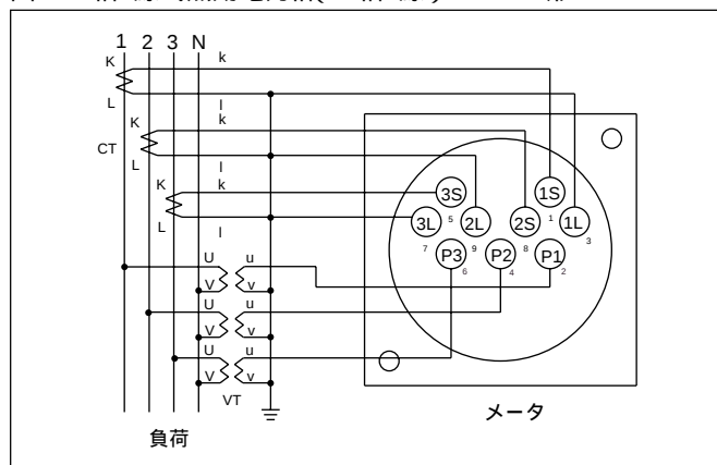
図4 三相4線式無効電力計(三相4線)SWC3-3形
