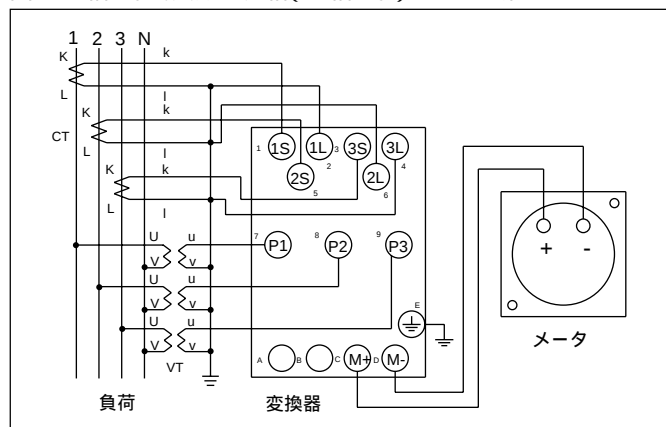
図3 三相4線式無効電力計(三相4線)SWC3-6形
