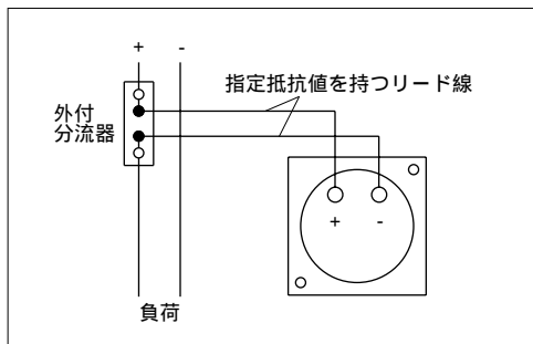
図2 直流電流計(分流器接続)
