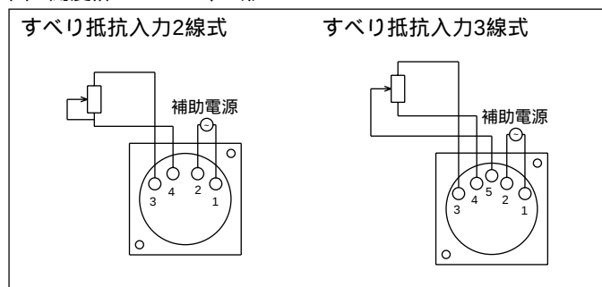
図5 開度計 SWMA-6、3形
